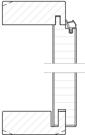
TF 51 Fase mit Einsatzfräsung
