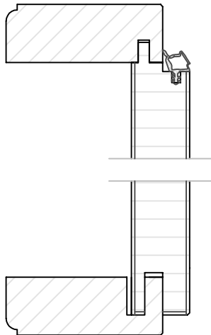
TF 54 Stabprofil
