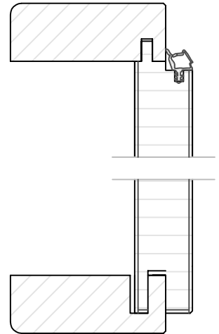
TF 53 Rundung 5mm
