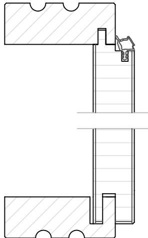
TF 55 Rillen (Aufpreis)
