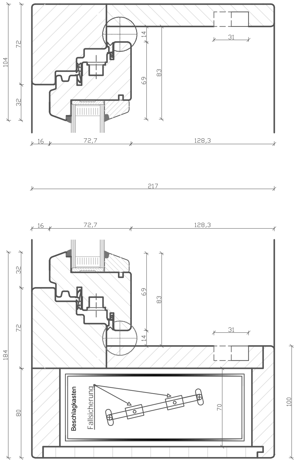
Systemzeichnung: Fallsicherung, unmaßstäblich
